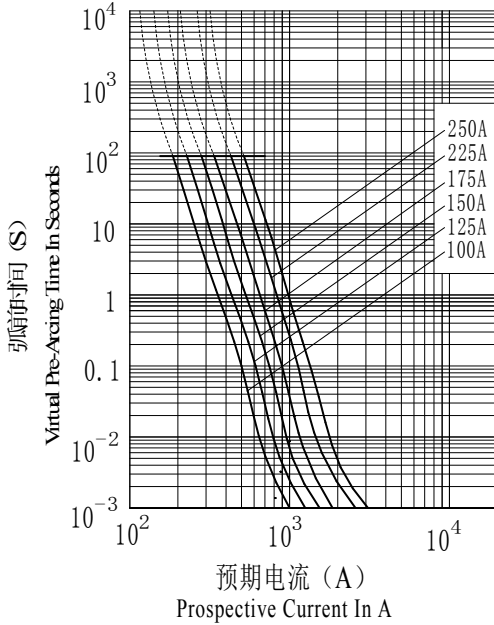
RS309-MD-EVS/EVS-D曲线
