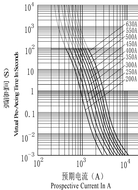
RS309-MD-EVS曲线
