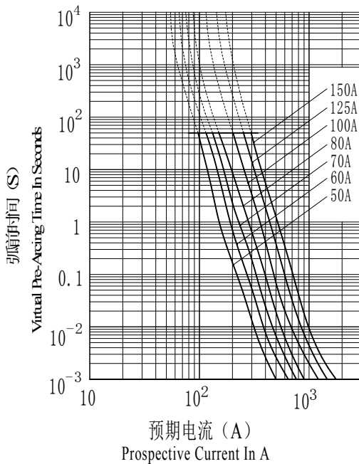
RS309-MD-EVS/EVS-D曲线
