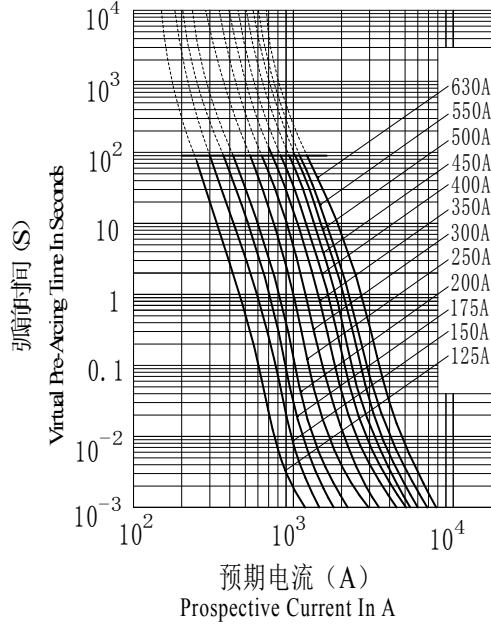
RS309-MD-EVS曲线
